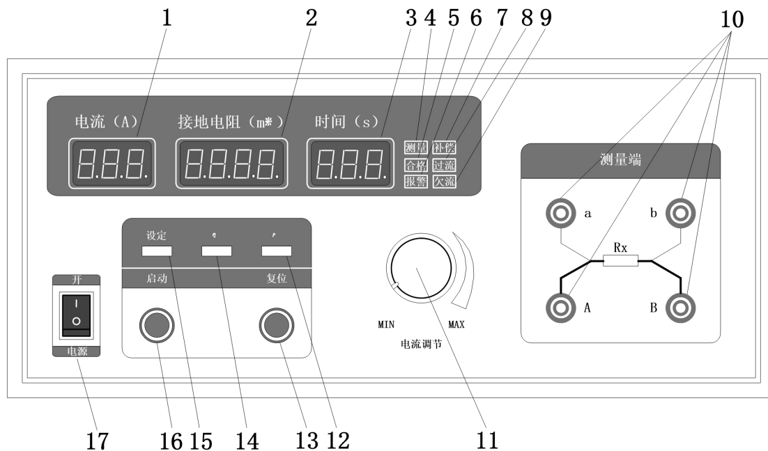
图 2 仪器面板
