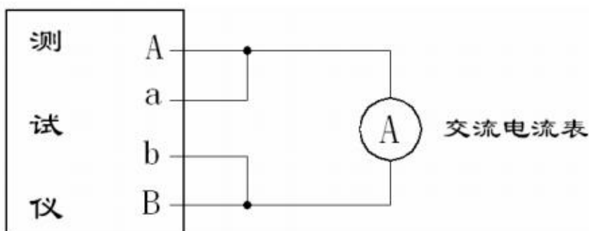
图 6 测试电流接线
