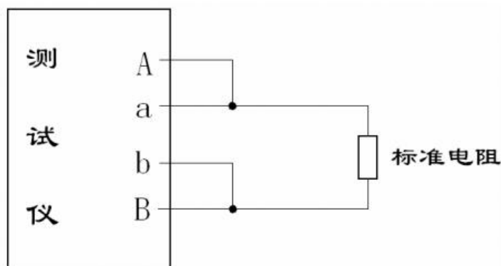
图 7 接地电阻接线
